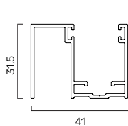
in allum. A32 41 x 31,5 mm GUAL..32M
