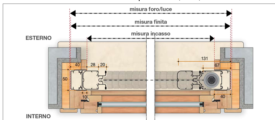
Sezione orizzontale 2 battenti con staffa attacco superiore con incasso 3 lati
