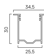
in allum. A34 25,5 x 30 mm GUAL..34M
