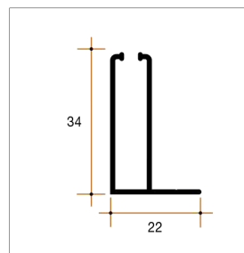
Cassonetto con barra maniglia e piastra
