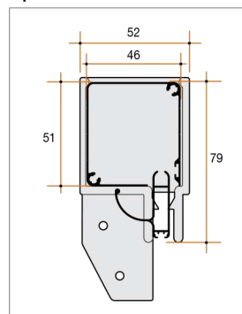
Cassonetto con barra maniglia e piastra
