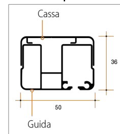
Guida telescopica
