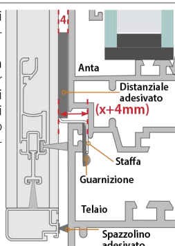
Serramento complanare
