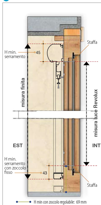
Serramento complanare
