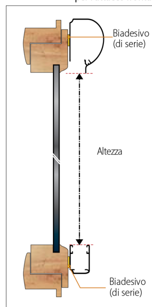
Rilevazione della misura vetro per l'attacco frontale
