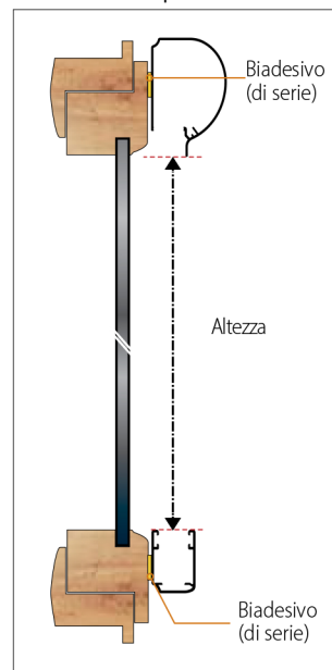
Rilevazione della misura vetro per l'attacco frontale
